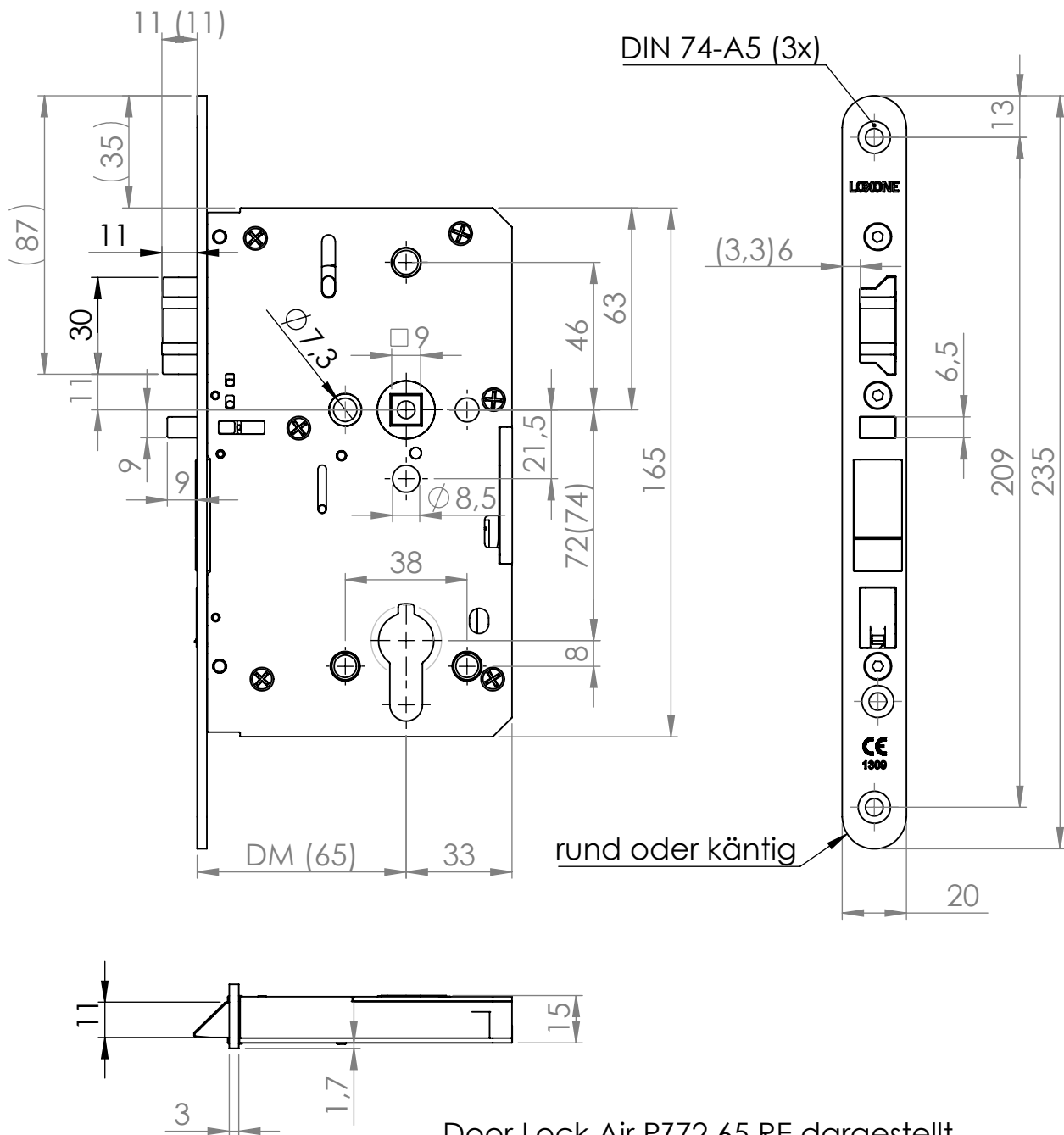
Door Lock Air PZ72 65 RE dargestellt Linksausführung spiegelbildlich
